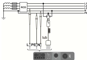
Pomiar w obwodzie L-PE
