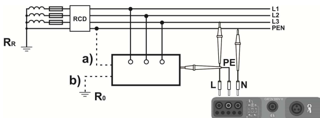
Sprawdzanie skuteczności ochrony przeciwporażeniowej obudowy urządzenia w przypadku: a) sieci TN b) sieci TT
