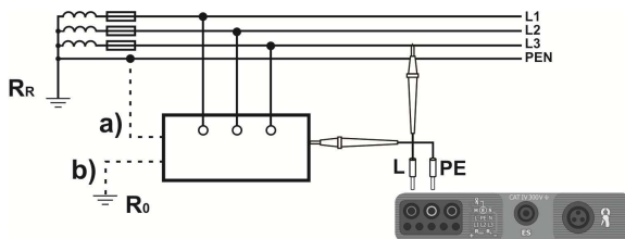
Sprawdzenie skuteczności ochrony przeciwporażeniowej obudowy urządzenia w przypadku: a) sieci TN b) sieci TT
